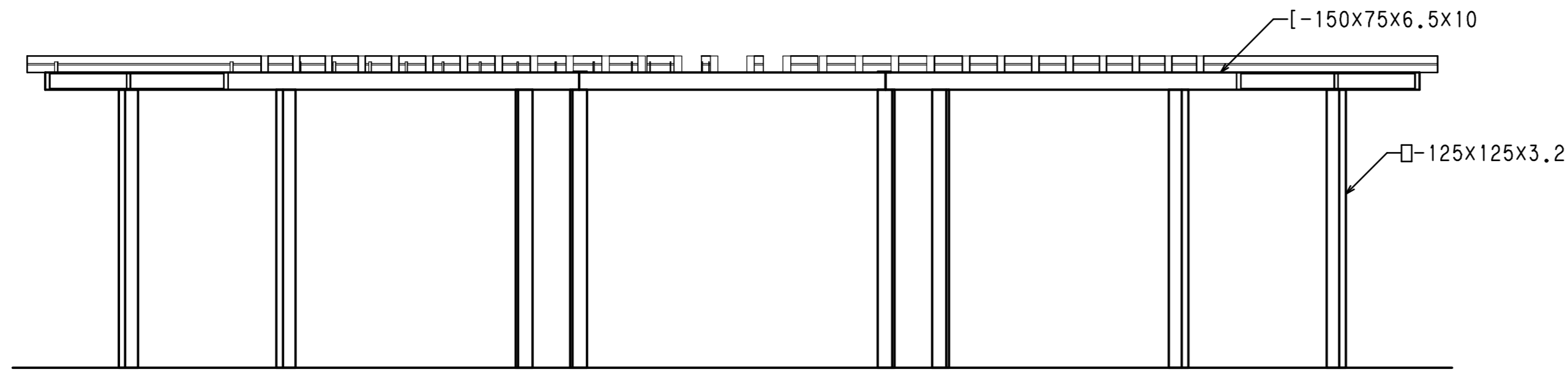
立面図 S=1/40
