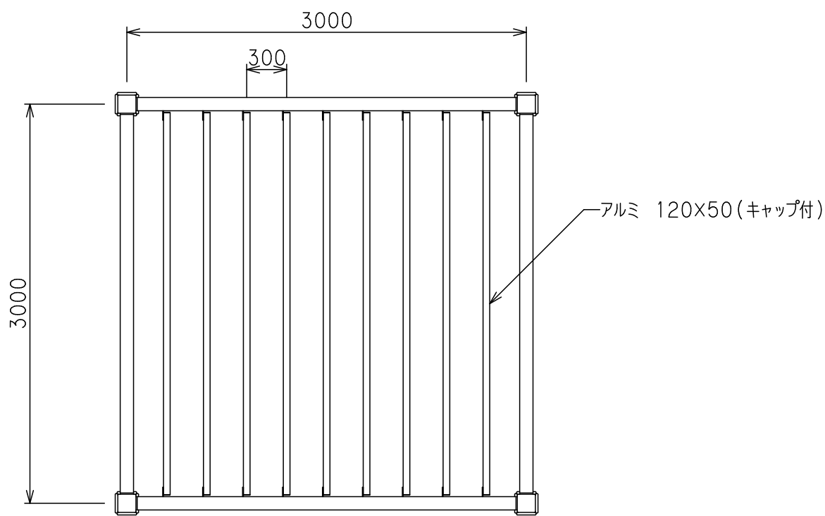
平面図 S=1/40
