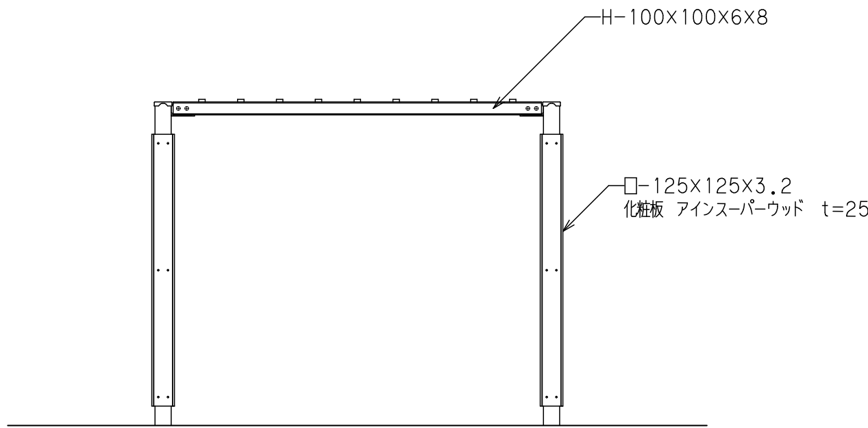
立面図 S=1/40
