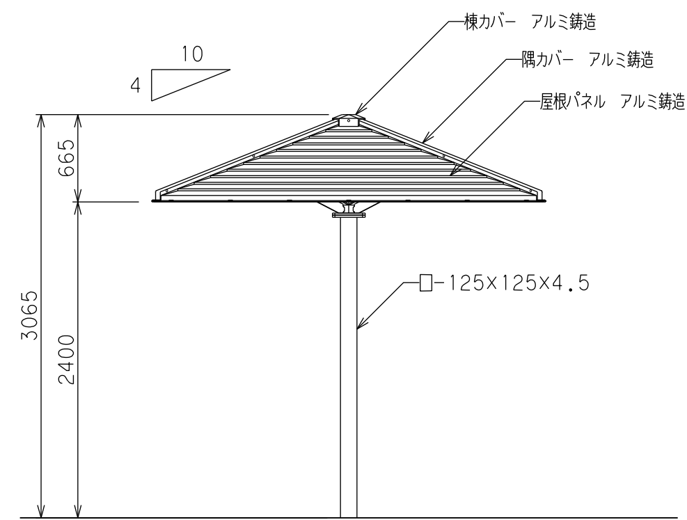
立面图 S=1/40
