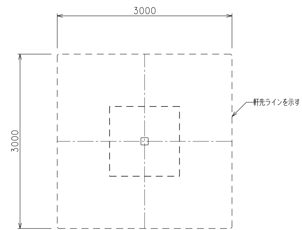
平面图 S=1/40
